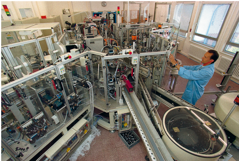
Mise en place de la ligne de fabrication initiale des microphones evolution
